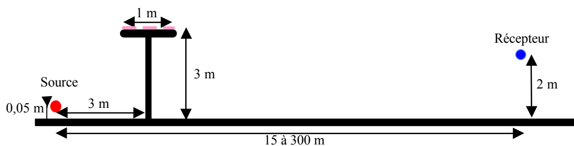
FIG. 2 – Géométrie de l'écran en T
