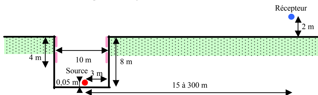
FIG. 3 – Géométrie de la tranchée
