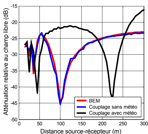
FIG. 5 – Atténuation par rapport au champ libre en fonction de la distance à la source pour une fréquence de 1000 Hz. Cas de l'écran en T (Fig. 2).
