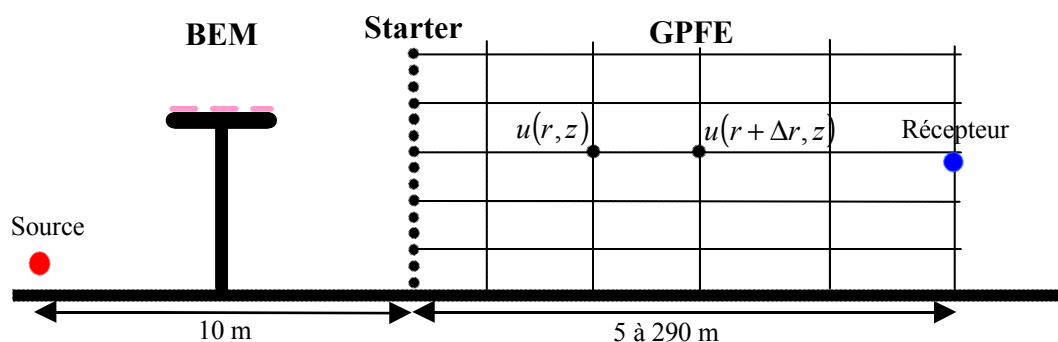
FIG. 4 – Configuration du couplage
