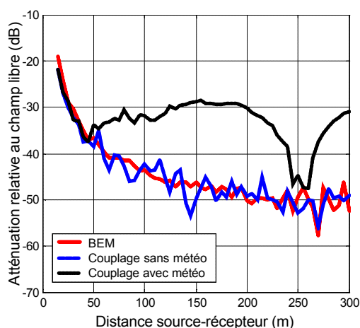
FIG. 6 – Atténuation par rapport au champ libre en fonction de la distance à la source pour une fréquence de 1000 Hz. Cas de la tranchée (Fig. 3).
